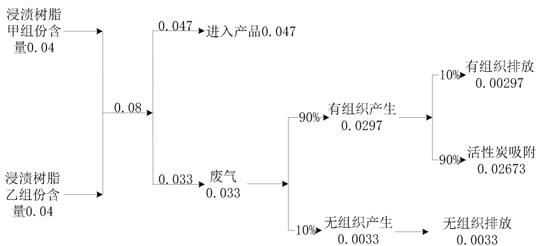
图 2-2 本项目苯系物（苯乙烯）平衡图 (t/a)
