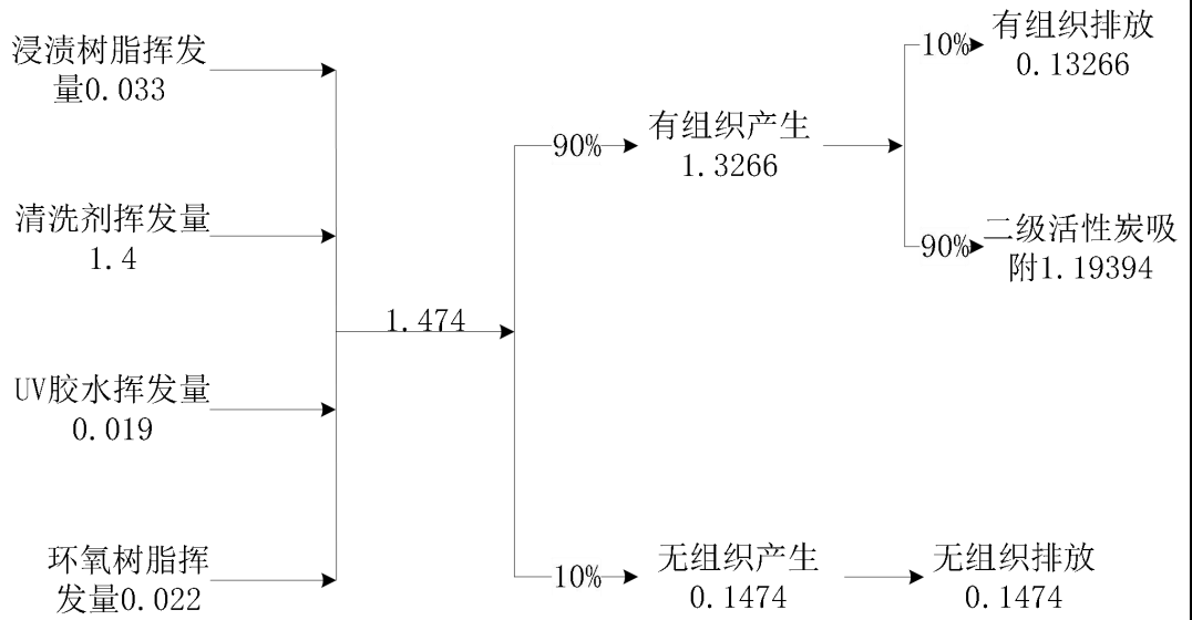
图 2-3 本项目 VOC（包含苯系物、非甲烷总烃）平衡图（t/a）
